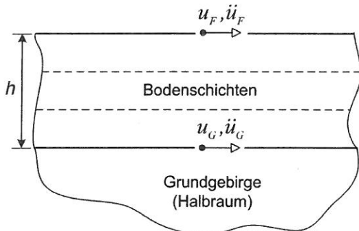
Bild 1. Bodenmodell für SH-Wellen Fig. 1. Soil model for SH waves
