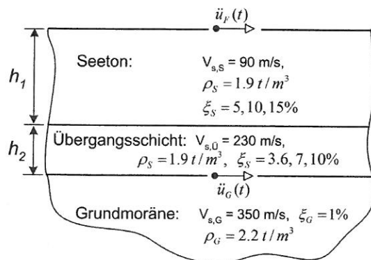
Bild 10. Zweischichtenmodell für Konstanzer Seeton Fig. 10. Two-layer model of Lake Constance clay
