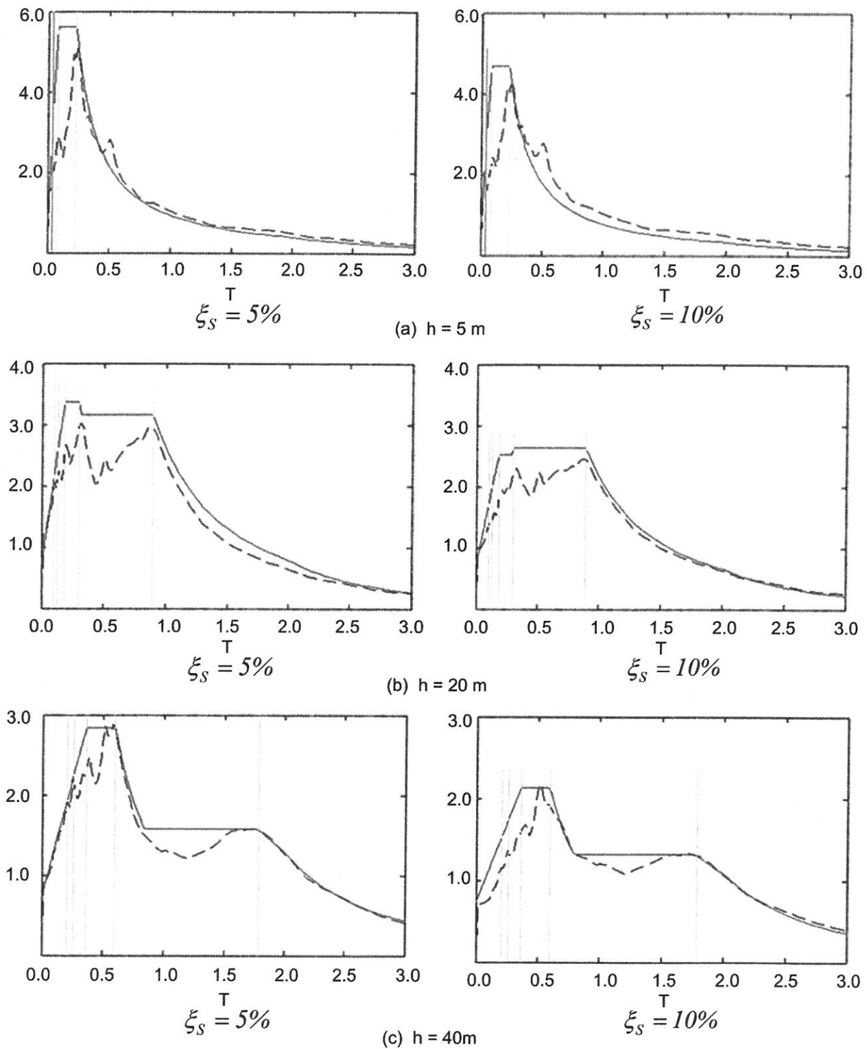
Bild 8. Vereinfachte horizontale Beschleunigungsantwortspektren für Konstanzer Seeton Fig. 8. Simplified horizontal acceleration response spectra for Lake Constance clay
