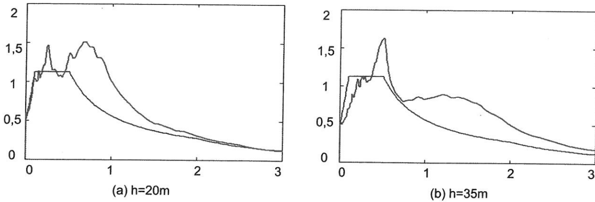
Bild 14. Äquivalente nichtlineare Berechnung eines Antwortspektrums, bezogen auf a_G = 0.6 \text{ m/s}^2 , \gamma_i = 1.0 , v_s = 115 \text{ m/s} Fig. 14. CEquivalent nonlinear computation of a response spectrum for a_G = 0.6 \text{ m/s}^2 , \gamma_i = 1.0 , v_s = 115 \text{ m/s}
