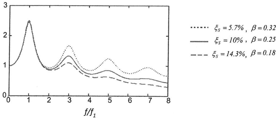
Bild 3. Übertragungsfunktionen |F(\Omega)| für SH-Wellen, Anpassung an die erste Resonanzstelle Fig. 3. Transfer function |F(\Omega)| for SH waves, adjustment of the first resonance peak
