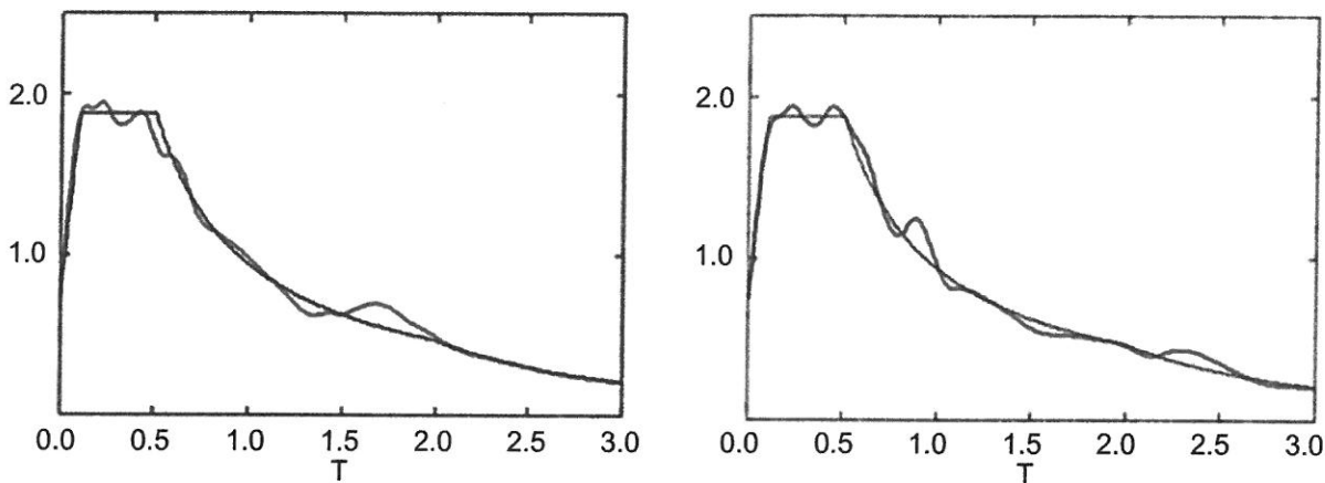
Bild 4. Antwortspektren zweier künstlicher Beschleunigungszeitverläufe \ddot{u}_G(t) auf der Grundmoräne Fig. 4. Response spectra of two artificially generated earthquake time histories \ddot{u}_G(t) on bedrock
