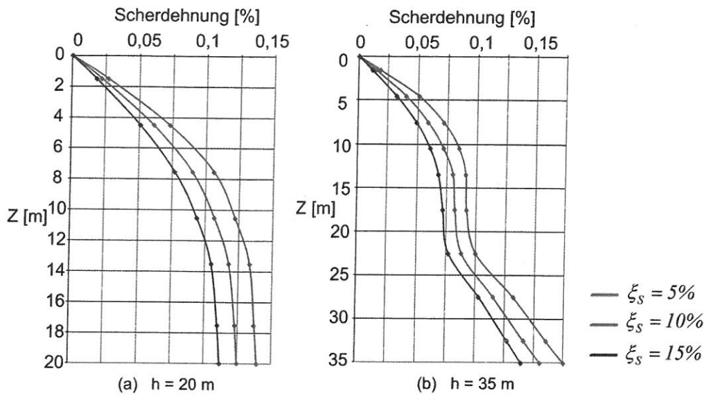
Bild 12. Maximale Scherdehnungen aufgetragen über die Schichthöhe, normiert auf a_G = 1.0 \text{ m/s}^2 , \gamma_I = 1.0 . Fig. 12. Maximum shear strains plotted with respect to depth for a_G = 1.0 \text{ m/s}^2 , \gamma_I = 1.0 .
