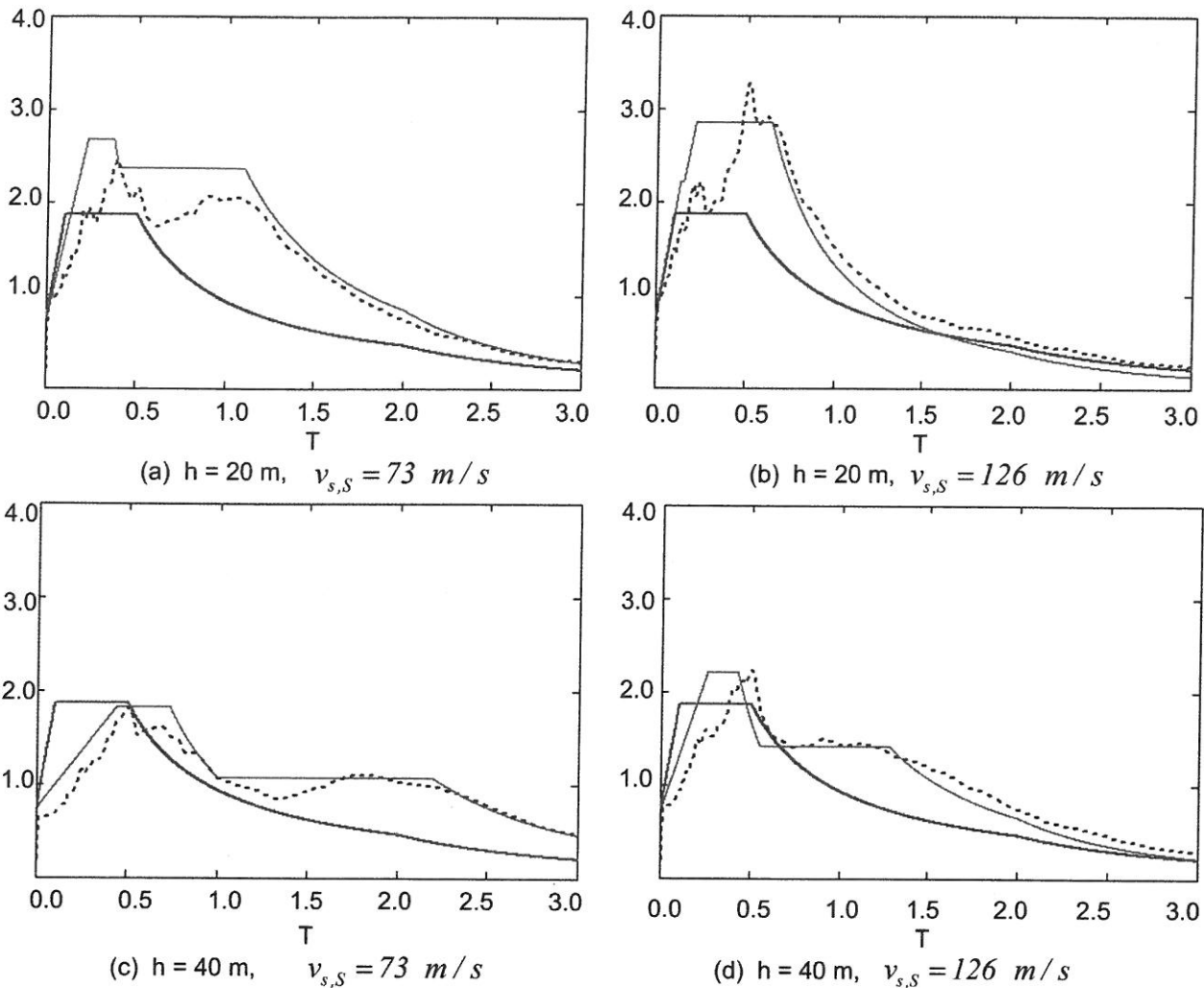
Bild 9. Näherungsweise Ermittlung von Beschleunigungsantwortspektrern, \xi_S = 10\% , normiert auf a_G = 1.0 \text{ m/s}^2, \gamma_I = 1.0 Fig. 9. Approximated determination of acceleration response spectra, \xi_S = 10\% for a_G = 1.0 \text{ m/s}^2, \gamma_I = 1.0
