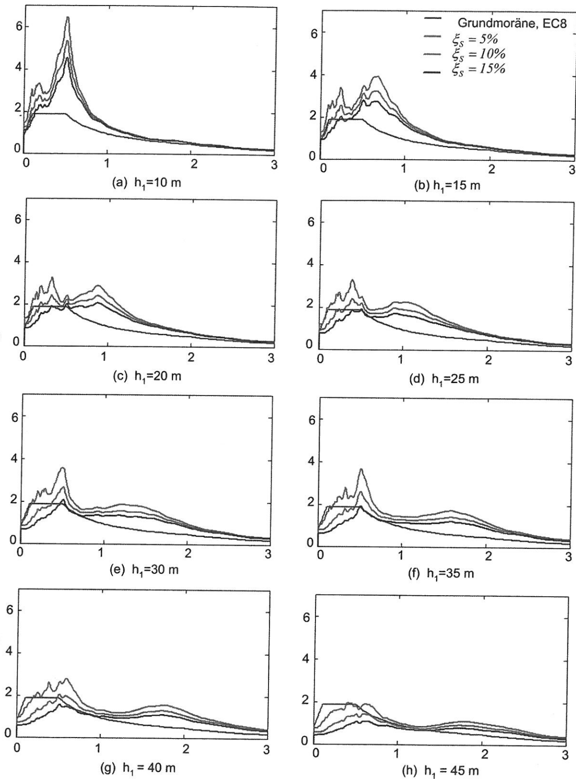
Bild 11. Horizontale Beschleunigungsantwortspektra für Konstanzer Seeton – Zweischichtenmodell, h_2 = 5 m, normiert auf a_G = 1.0 \text{ m/s}^2 , \gamma_I = 1.0
