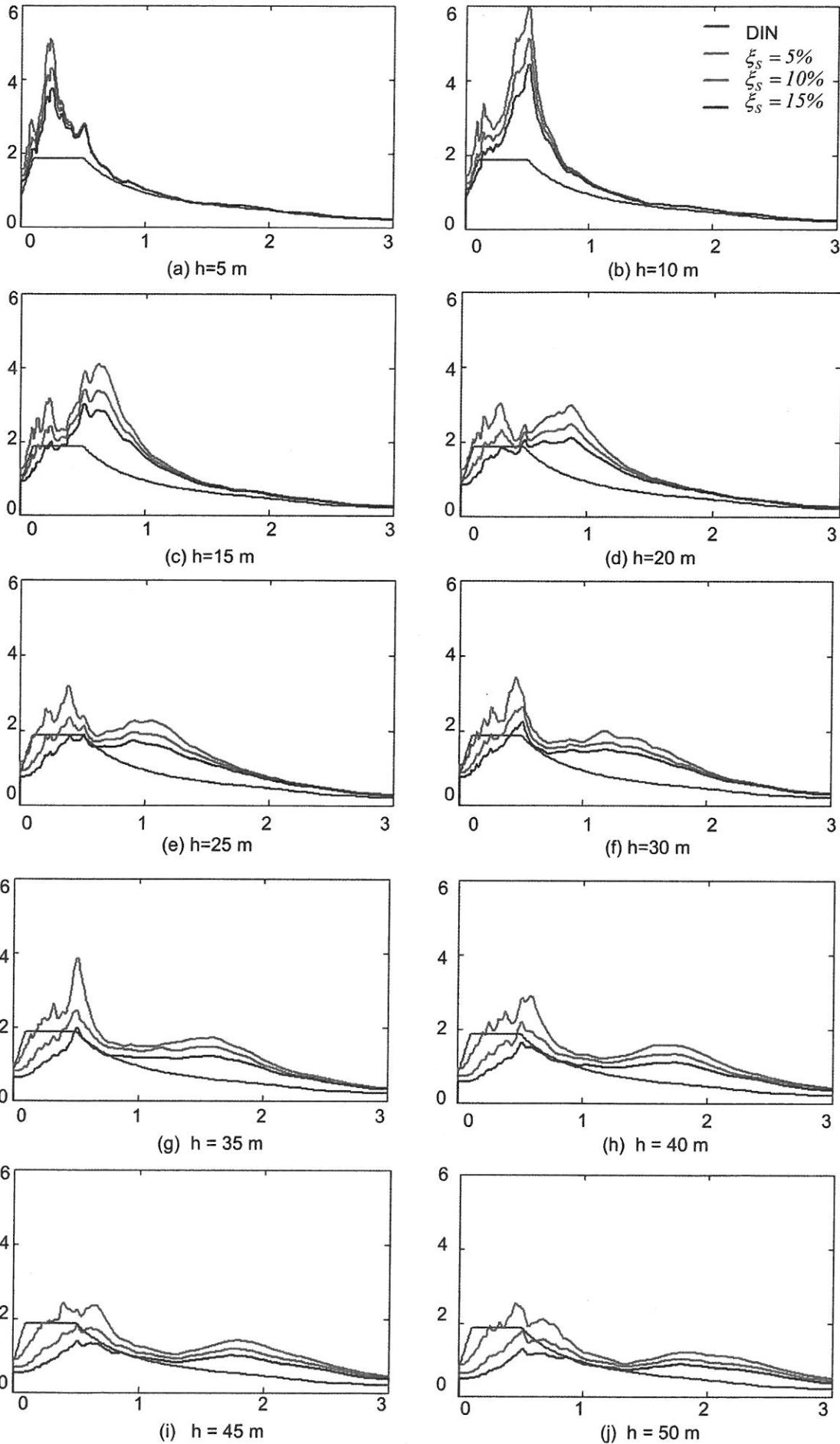
Bild 6. Horizontale Beschleunigungsantwortspektra für Konstanzer Seeton, normiert auf a_G = 1.0 \text{ m/s}^2 , \gamma_I = 1.0 Fig. 6. Horizontal acceleration response spectra for Lake Constance clay, for a_G = 1.0 \text{ m/s}^2 , \gamma_I = 1.0
