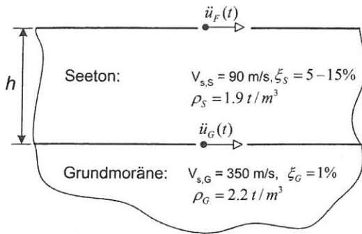
Bild 5. Einschichtmodell für Konstanzer Seeton Fig. 5. One-layer model for clay deposits of the Lake Constance area
