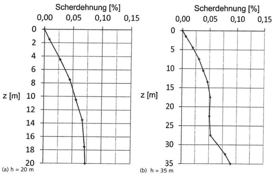
Bild 13. Äquivalente nichtlineare maximale Scherdehnungen, bezogen auf a_G = 0.6 \text{ m/s}^2 , \gamma_I = 1.0 , v_s = 115 \text{ m/s} . Fig. 13. Equivalent maximum shear strains plotted with respect to depth for a_G = 0.6 \text{ m/s}^2 , \gamma_I = 1.0 , v_s = 115 \text{ m/s} .
